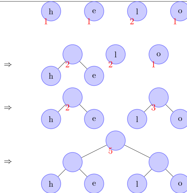
FIG. 2 – Construction d'un arbre de Huffman
