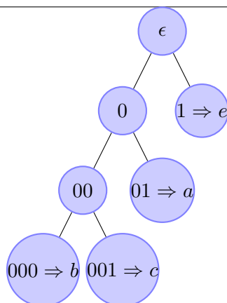
FIG. 1 – Arbre de Huffman
